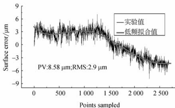
图 19 掠入射反射镜面形初始误差
