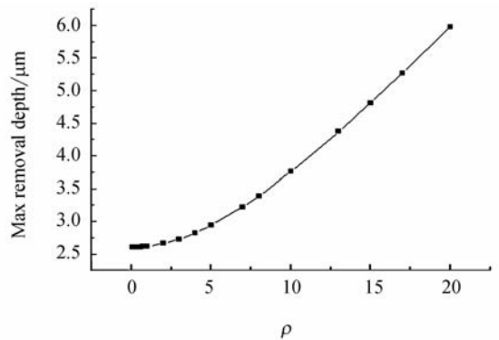
图 7 \rho 对去除函数的影响
