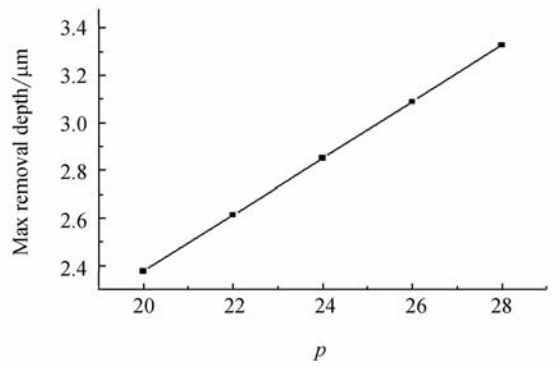
图 10 中心压力 p_0 对去除函数的影响
