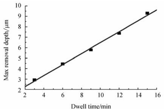
图 11 去除函数的中心去除深度与驻留时间的关系
