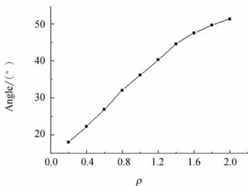
图 18 \rho 与速度轨迹方向-Y轴夹角关系图
