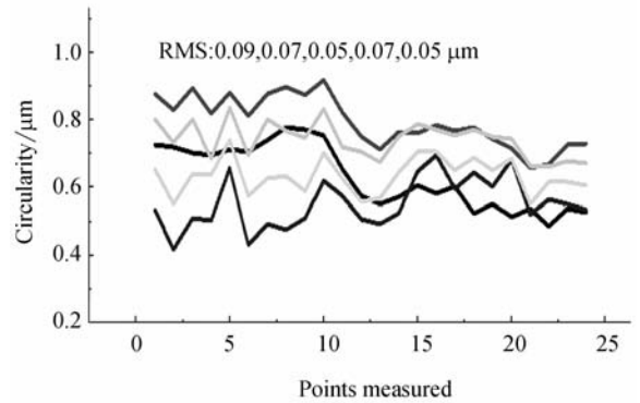
图26 掠入射反射镜圆度误差分布
