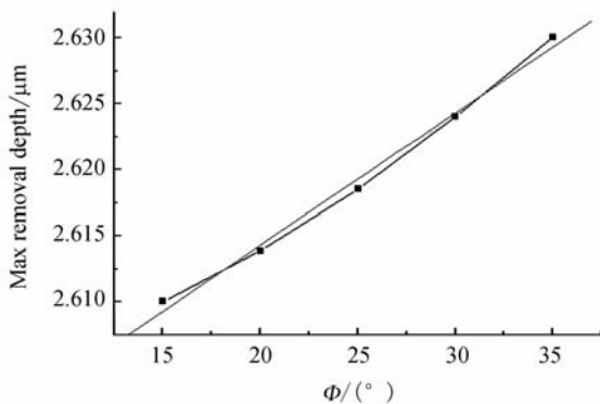
图 9 旋偏角对去除函数的影响
