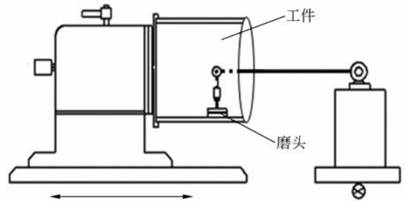
图 1 Wolter I 型掠入射反射镜数控研抛机
