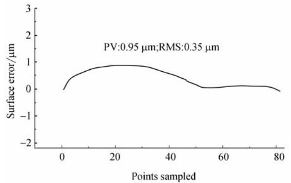
图 23 三次迭代加工后的面形误差
