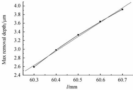
图 8 l 对去除函数的影响
